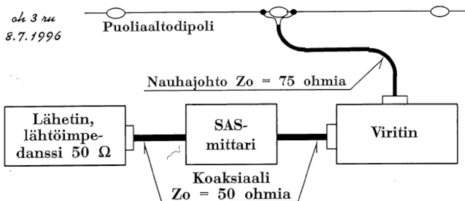
Lähettimen virittäminen antenniin
